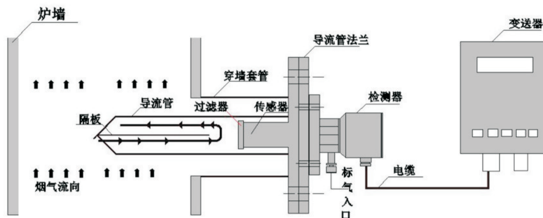
高温导流式氧化锆氧量分析仪安装示意图 使用温度：0-1200 ^{\circ}\text{C}
